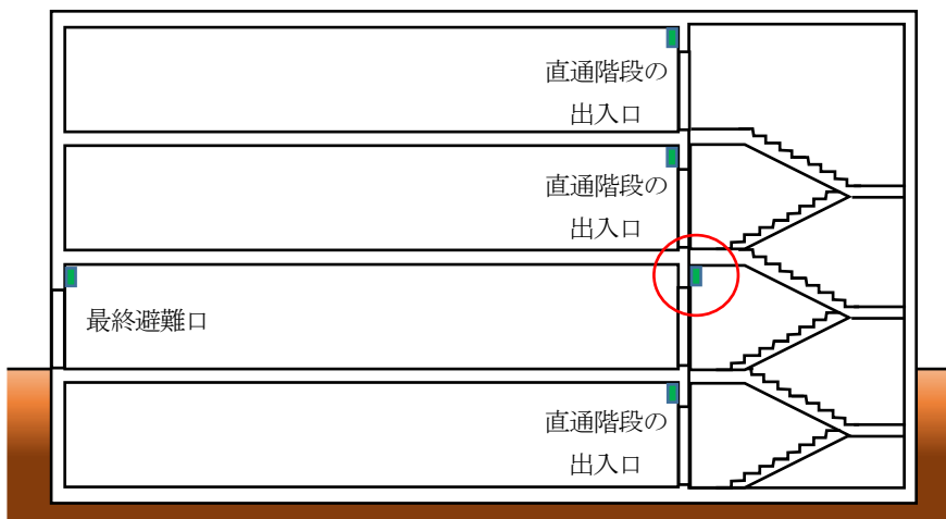
（立面図）
