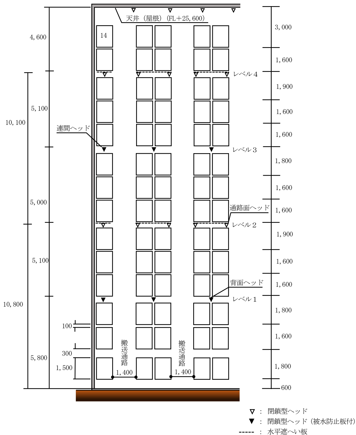
(断面図)
